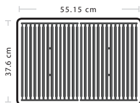
Ruszty Żeliwne SERIA MONARCH™
